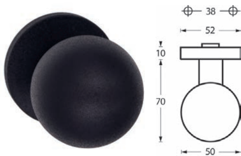
543-21 / vast Hartafstand: 38 mm Ø rozet: 52 mm Ø knop: 50 mm alleen bij vleugeloverdekkend paneel mogelijk! (montage op paneel)
